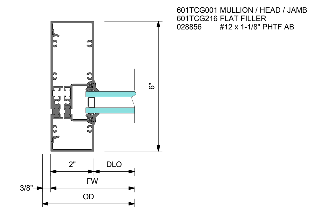
4 DETAIL 4 JAMB
