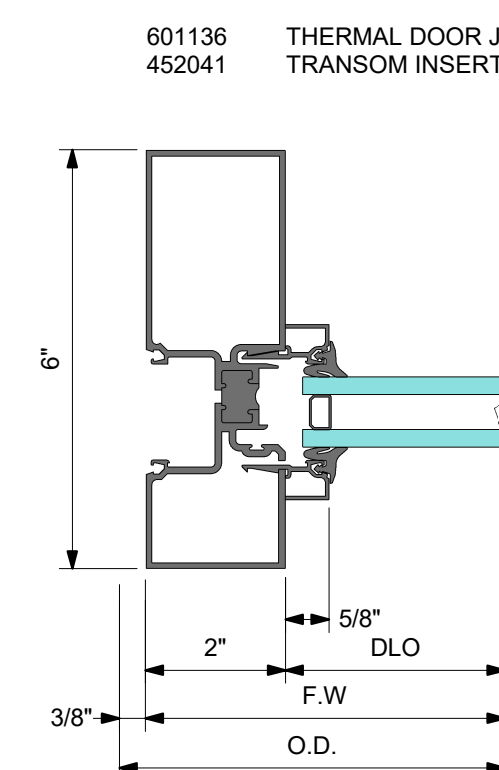
4A DETAIL 4A TRANSOM JAMB
