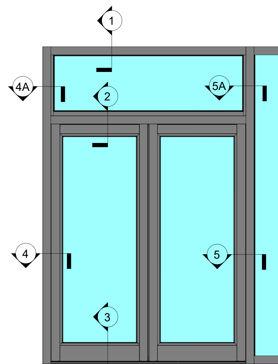
ELEVATION
