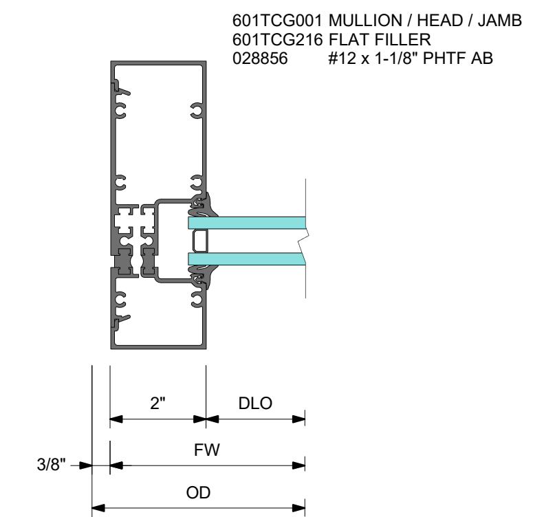
4 DETAIL 4 JAMB
