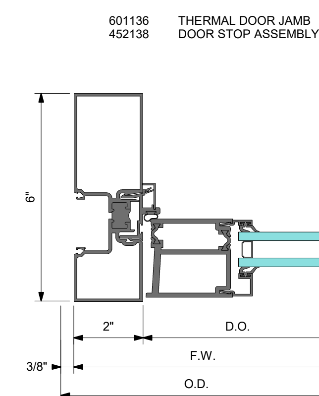
4 DETAIL 4 DOOR JAMB
