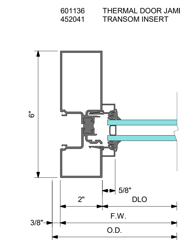
4A DETAIL 4A TRANSOM JAMB
